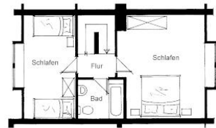
Grundriß Dachgeschoß
